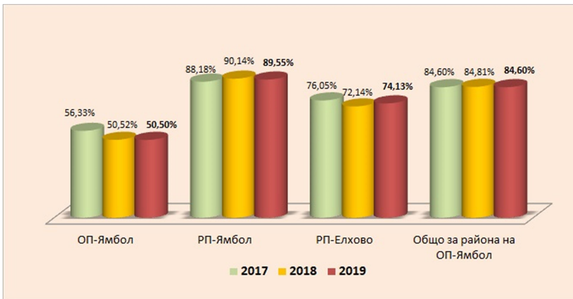
фиг.8 Относителен дял на решените от наблюдаваните ДП по години и прокуратури
