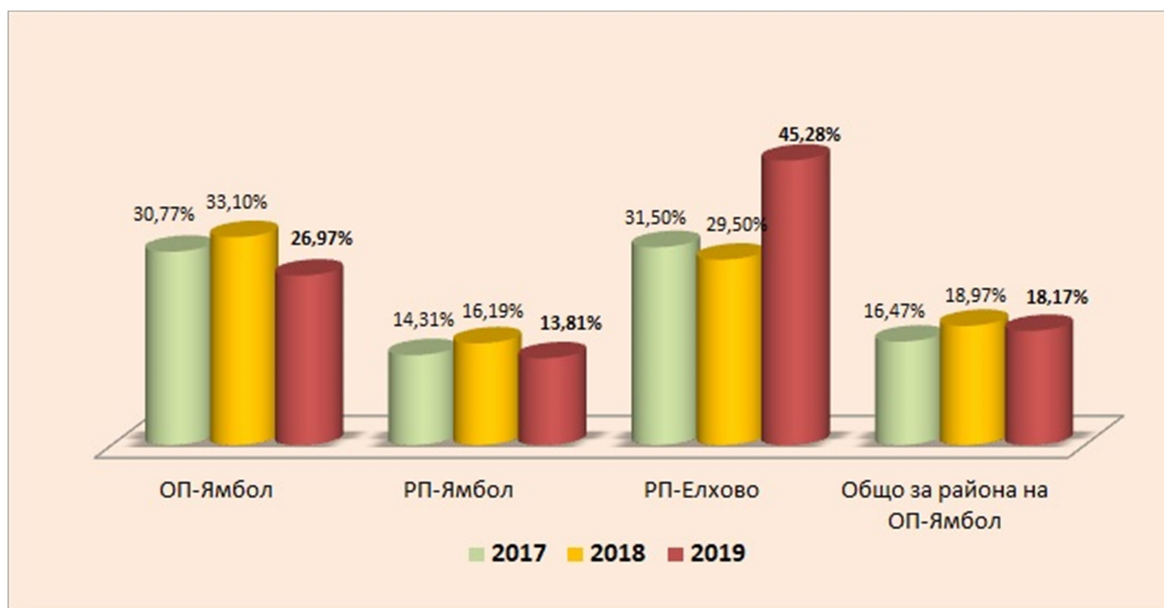
фиг.10 Относителен дял на внесените в съда от решените ДП по години и прокуратури
