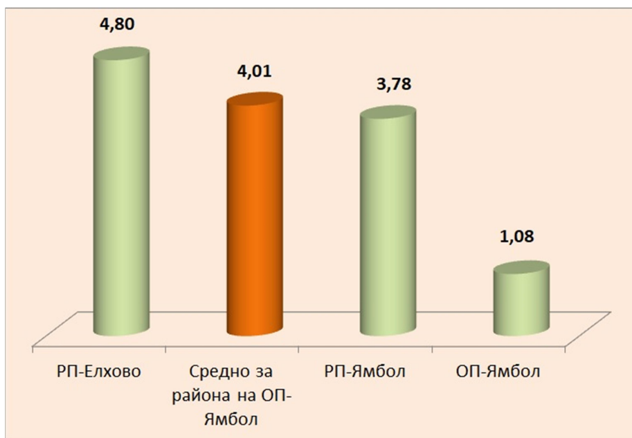
фиг.36 Средна натовареност на един прокурор в прокуратурите от съдебния район на ОП-Ямбол (брой точки на ден)
