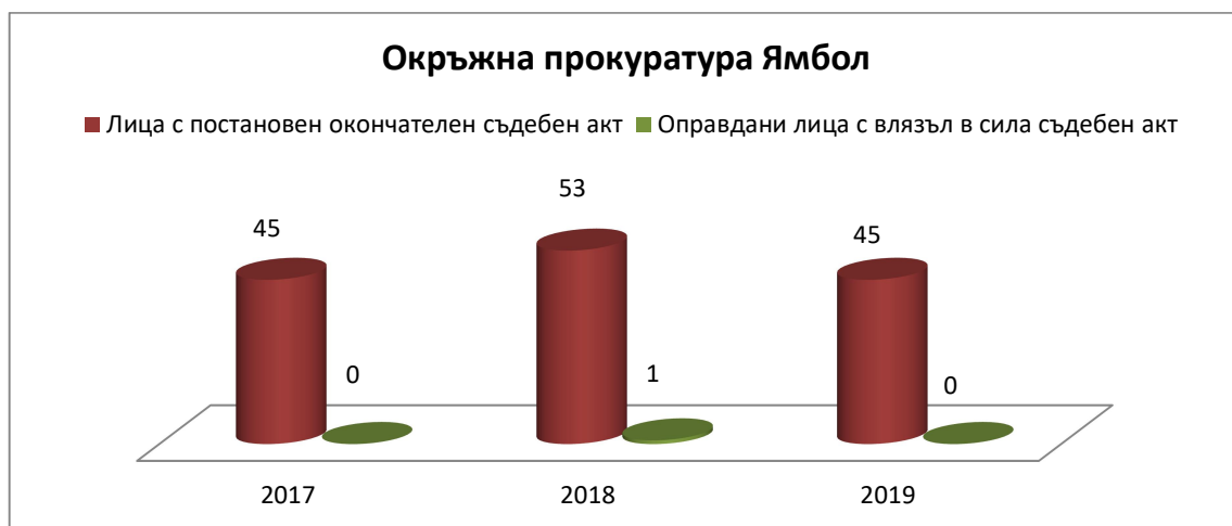
фиг.27 Относителен дял на оправданите с влязъл в сила съдебен акт лица от всички с постановен окончателен съдебен акт за Окръжна прокуратура Ямбол
