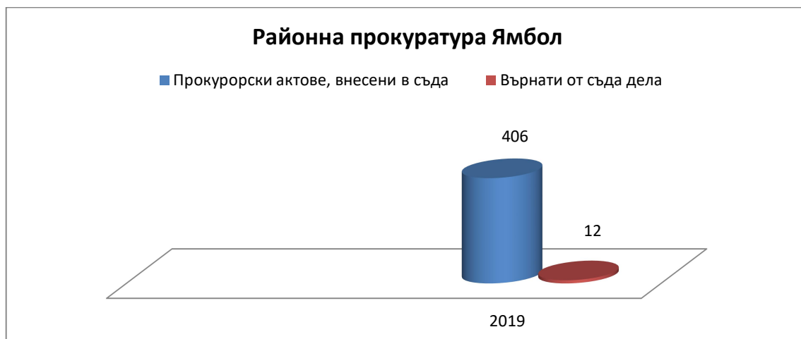
фиг.16 Внесени в съда прокурорски актове и върнати от съда дела на прокуратурата в абсолютни стойности за Районна прокуратура Ямбол
