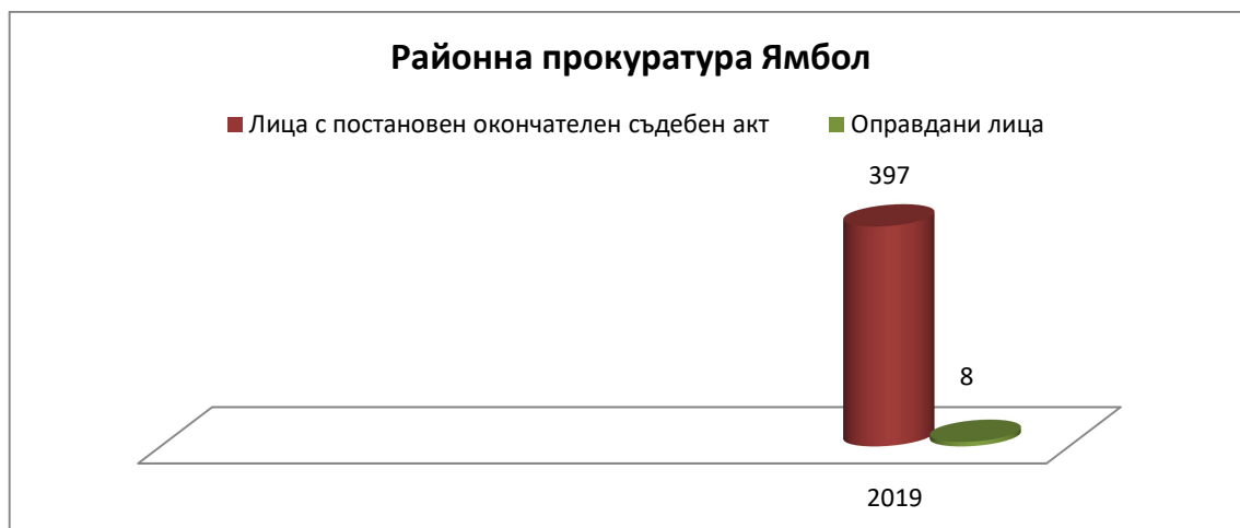
фиг.24 Относителен дял на оправданите лица от всички с постановен окончателен съдебен акт за Районна прокуратура Ямбол
