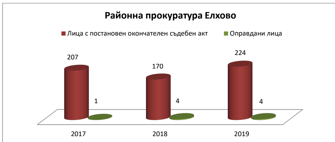
фиг.25 Относителен дял на оправданите лица от всички с постановен окончателен съдебен акт за Районна прокуратура Елхово
