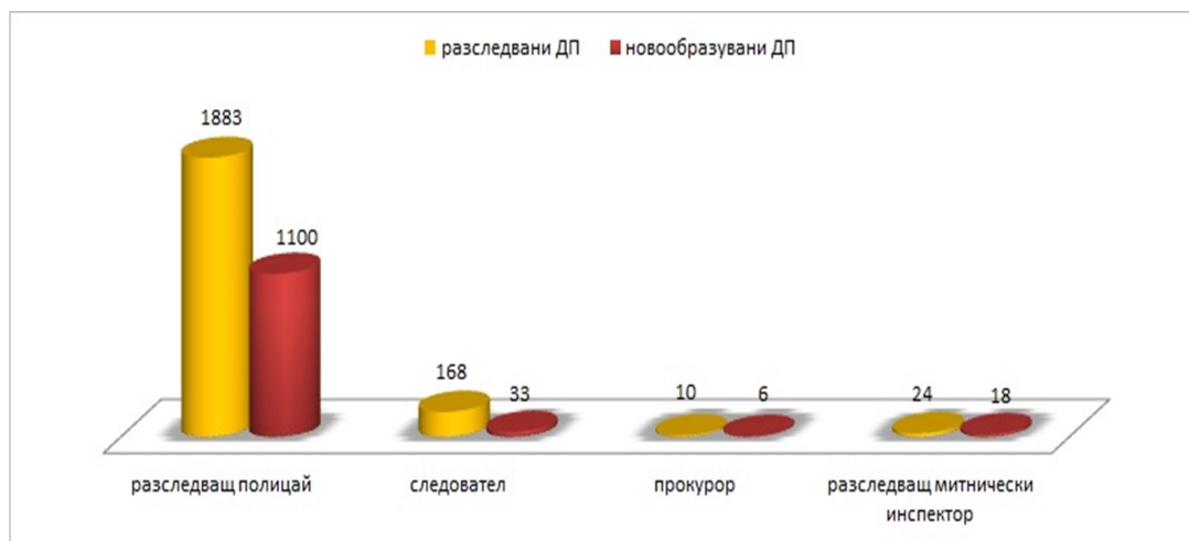
фиг.5 Брой разследвани ДП и новообразуваните от тях, по видове разследващи органи
