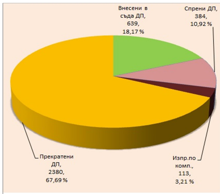
фиг.9 Решени ДП през 2019 г.
