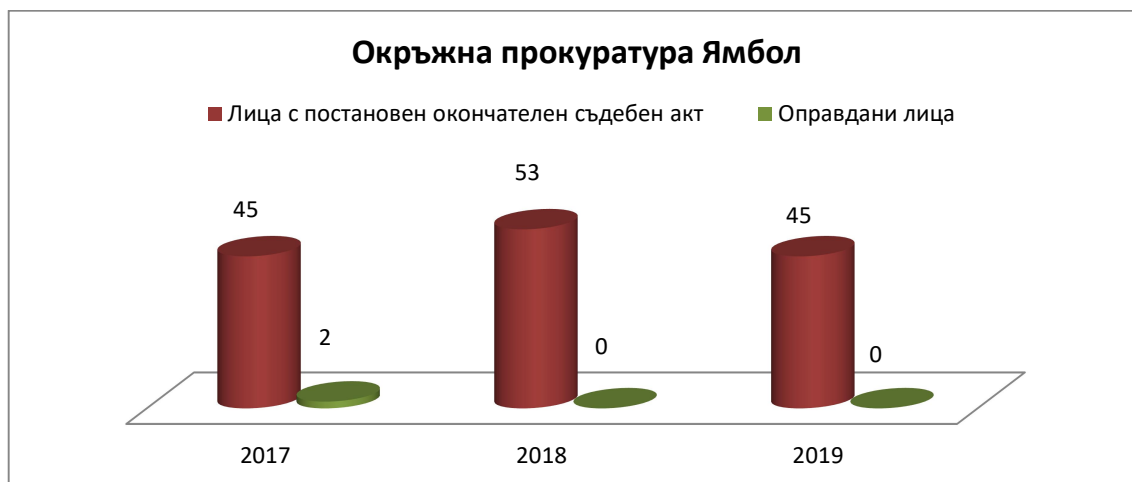
фиг.23 Относителен дял на оправданите лица от всички с постановен окончателен съдебен акт за Окръжна прокуратура Ямбол
