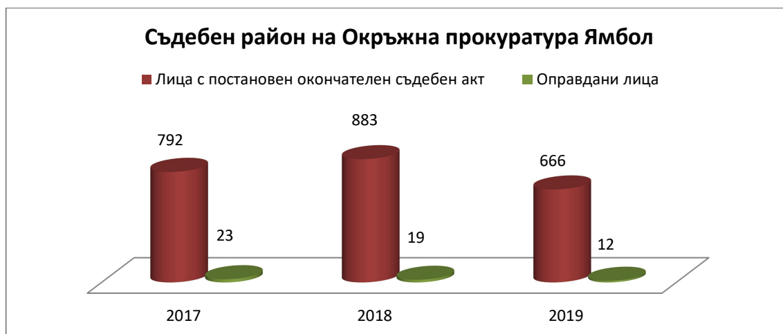
фиг.22 Относителен дял на оправданите лица от всички с постановен окончателен съдебен акт за съдебния район на Окръжна прокуратура Ямбол
