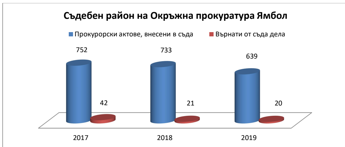
фиг.14 Внесени в съда прокурорски актове и върнати от съда дела на прокуратурата в абсолютни стойности за съдебния район на Окръжна прокуратура Ямбол
