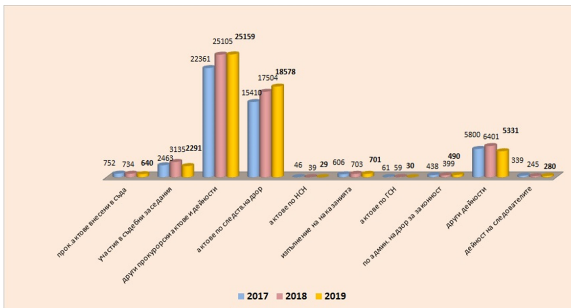
фиг.33 Обем и средна натовареност в ОП-Ямбол през последните три години
