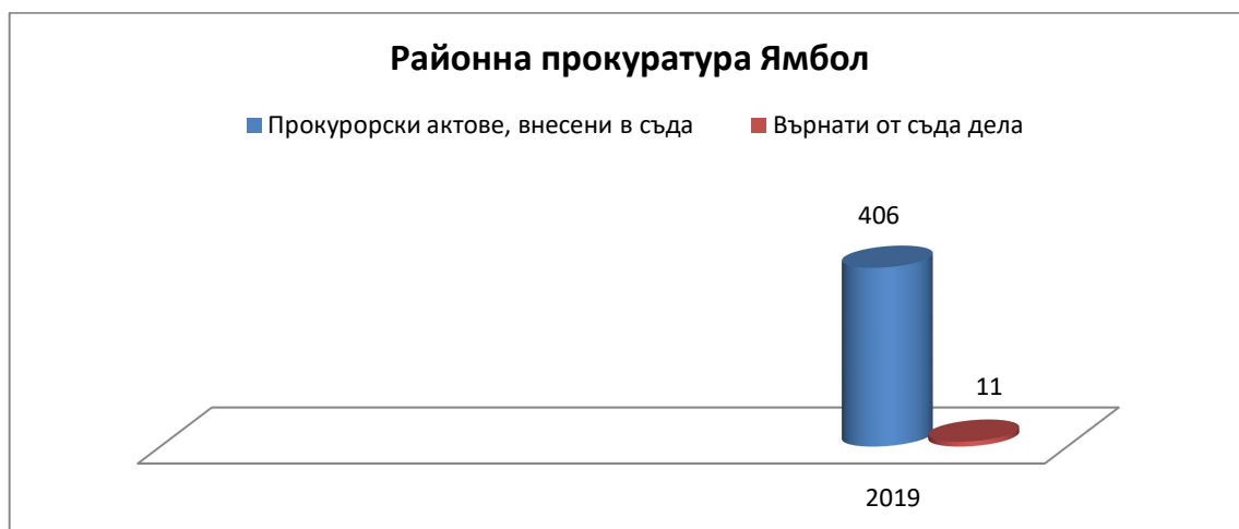
фиг.20 Внесени в съда прокурорски актове и върнати от съда дела на прокуратурата в абсолютни стойности за съдебния район на Районна прокуратура Ямбол
