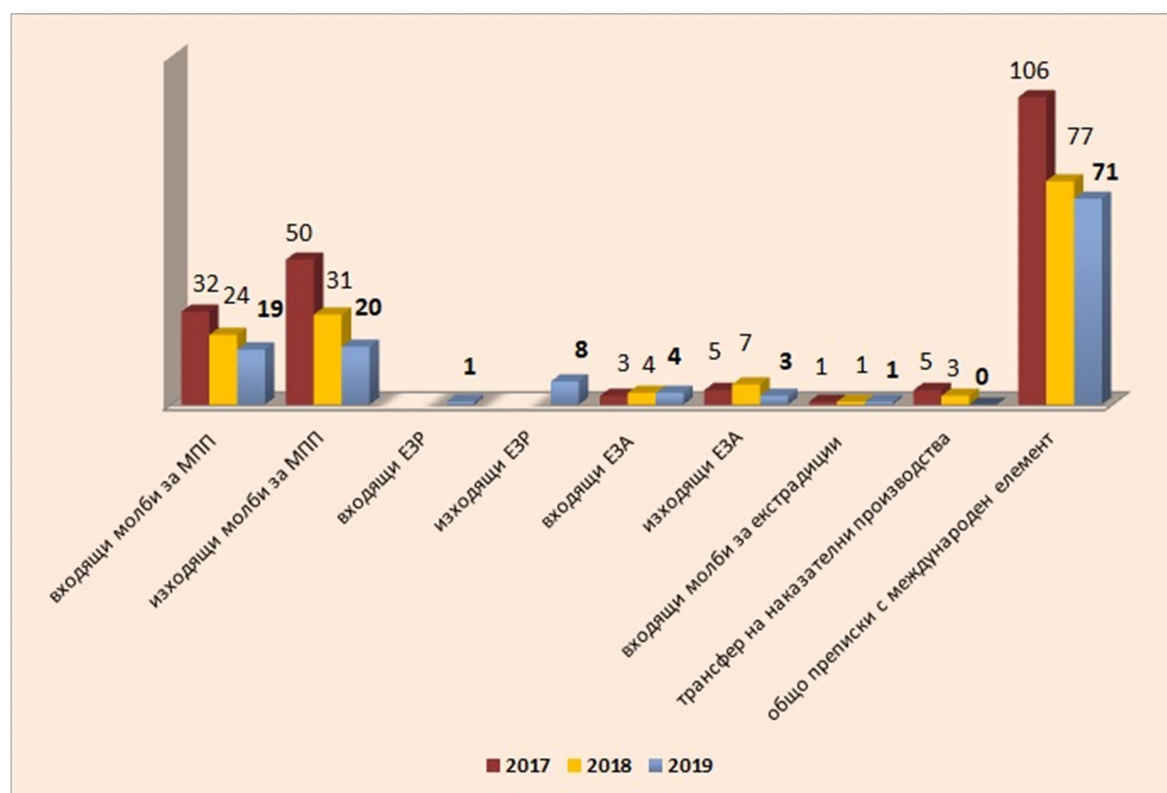
фиг.31 Дейност по международно правно сътрудничество през последните три години
