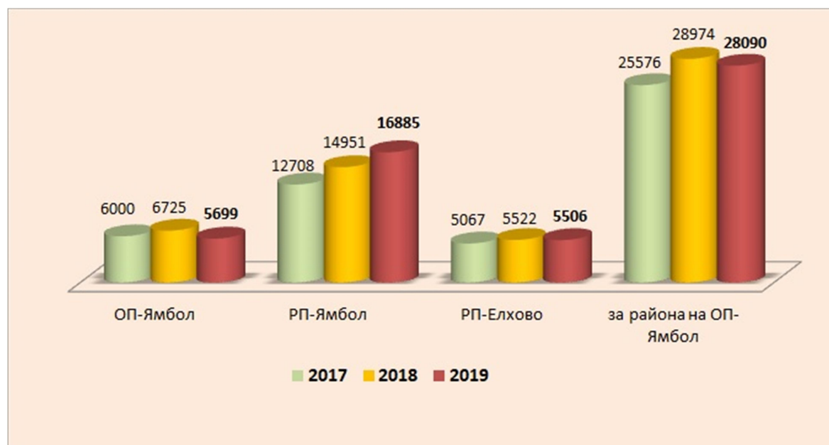
фиг.32 Общ обем на прокурорската дейност за последните три години
