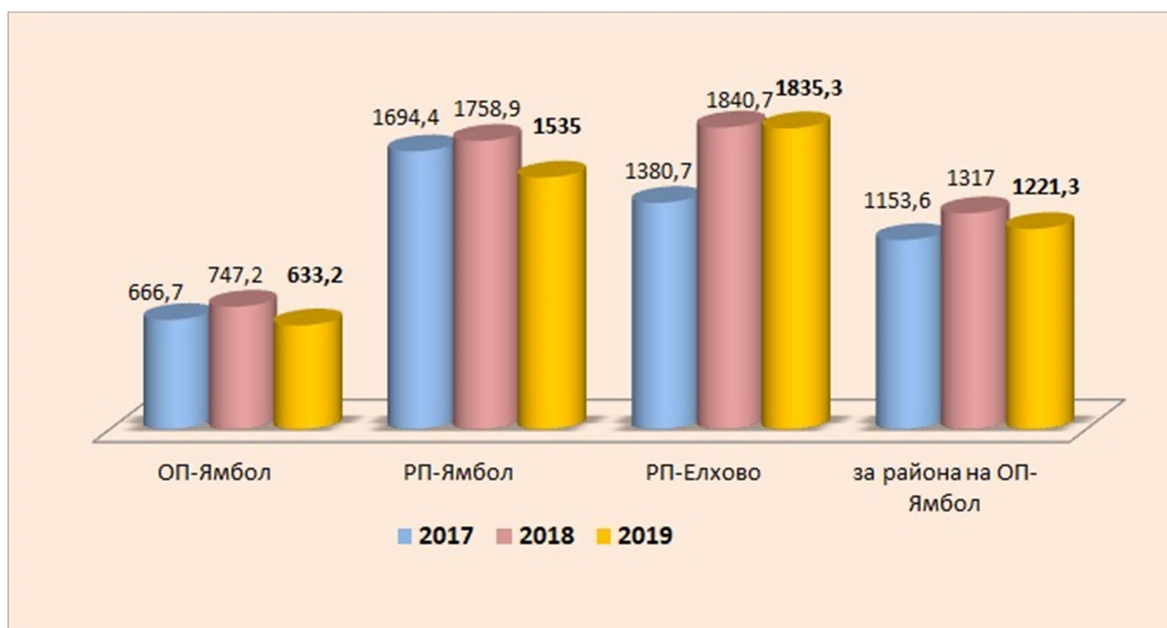
фиг.34 Средна натовареност на един прокурор
