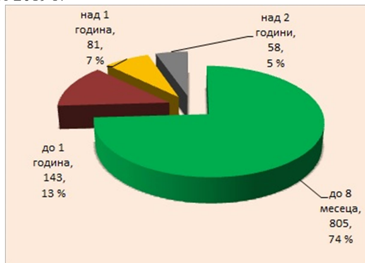
фиг.7 Продължителност на досъдебната фаза по приключени и решени ДП с прекратяване или внасяне в съда през 2019 г.
