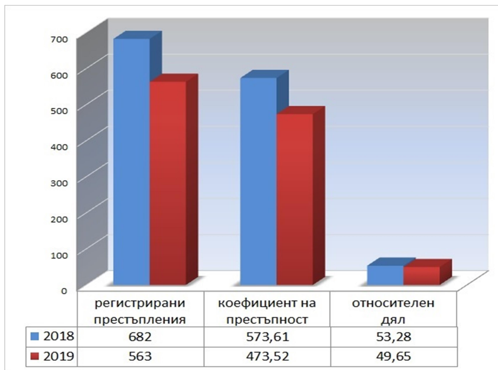
фиг.1 Регистрирани престъпления против собствеността, коефициент на престъпност и относителен дял
