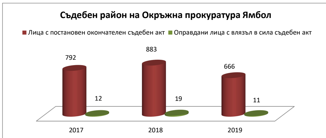
фиг.26 Относителен дял на оправданите с влязъл в сила съдебен акт лица от всички с постановен окончателен съдебен акт за съдебния район на Окръжна прокуратура Ямбол
