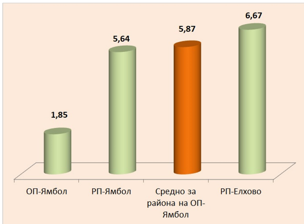
фиг.35 Средна натовареност на един прокурор в прокуратурите от съдебния район на ОП-Ямбол (брой актове на ден)
