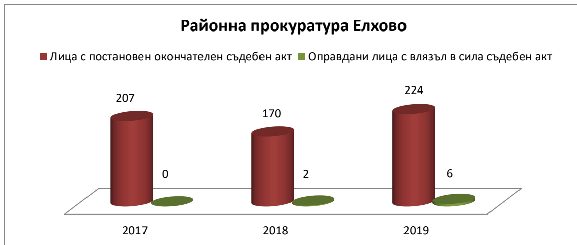
фиг.29 Относителен дял на оправданите с влязъл в сила съдебен акт лица от всички с постановен окончателен съдебен акт за Районна прокуратура Елхово
