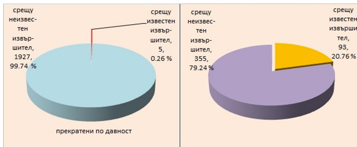
фиг.12 Относителен дял на прекратените ДП срещу известен и неизвестен извършител
